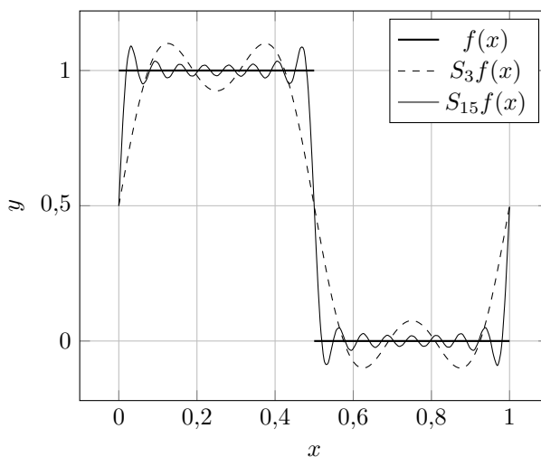
Slika 9.1: Graf prikazuje funkcijo f = \chi_{[0,1/2]} (z debelo), Fourierovo delno vsoto S_3 f(x) (z črtkano) in Fourierovo delno vsoto S_{15} f(x) (s polno). Razvidno je, da več členov v vrsti da boljši približek.
